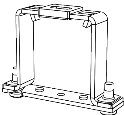
Věšák lišty horní mechanický - Fe profil P 002/32 (7-201862-0000) 56x58
